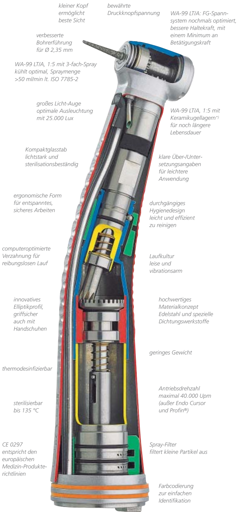
Bohrerwechsel auf Knopfdruck – einfacher geht's nicht!
